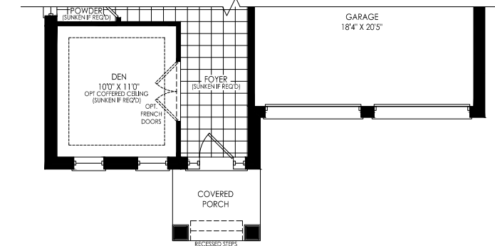
ELEVATION B
