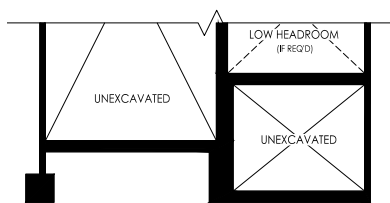
ELEVATION AC
